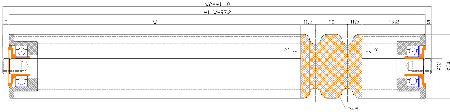
SECTION A-A'
